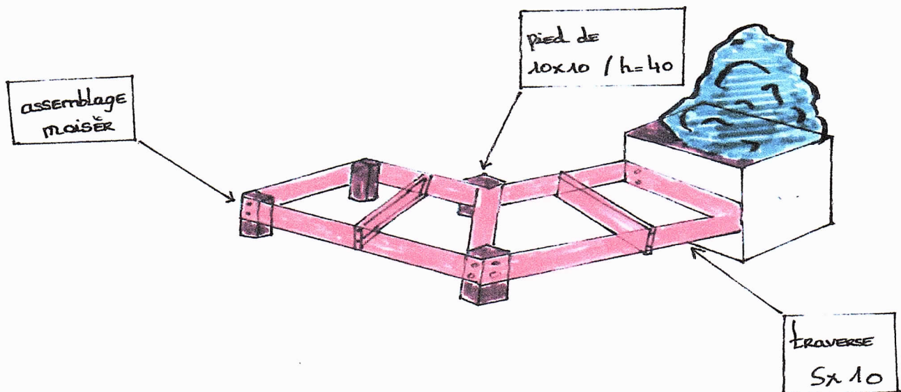
CROQUIS du Banc Jardinier
